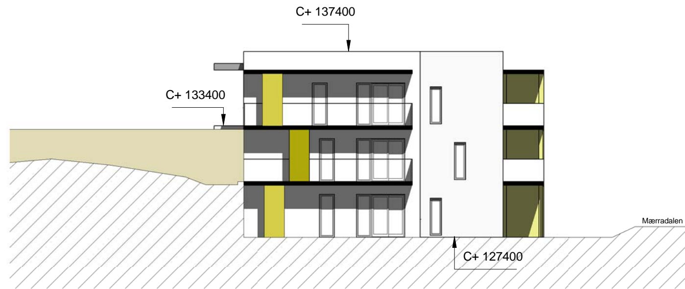
Fasade Øst
