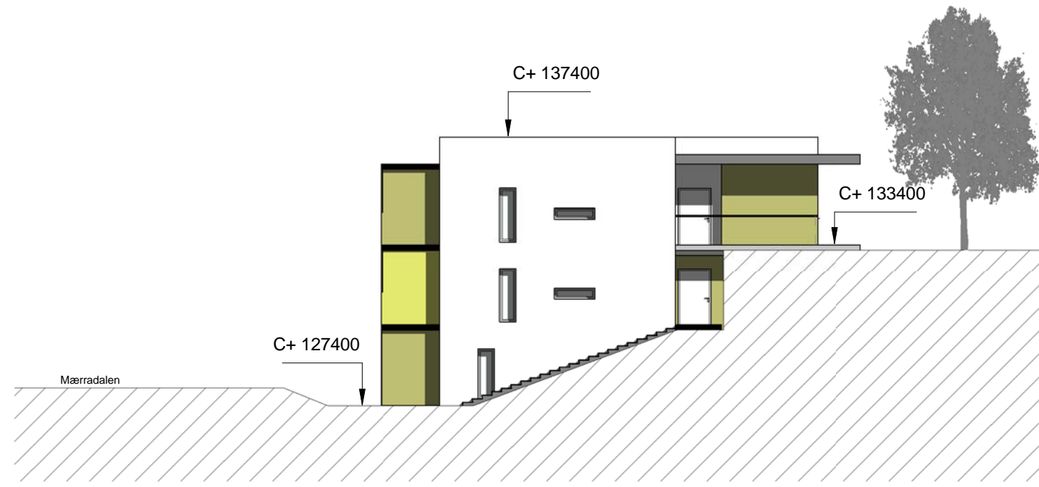
Fasade Vest
